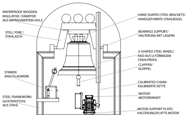
COMPLETE SWINGING BELL (VOLTEO) GLOCKE MIT ÜBERSCHLAG (VOLTEO)
