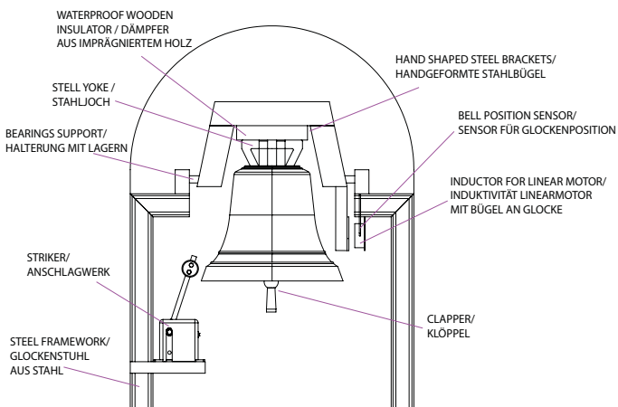
LINEAR MOTOR BELL SYSTEM GLOCKE MIT LINEARMOTOR
