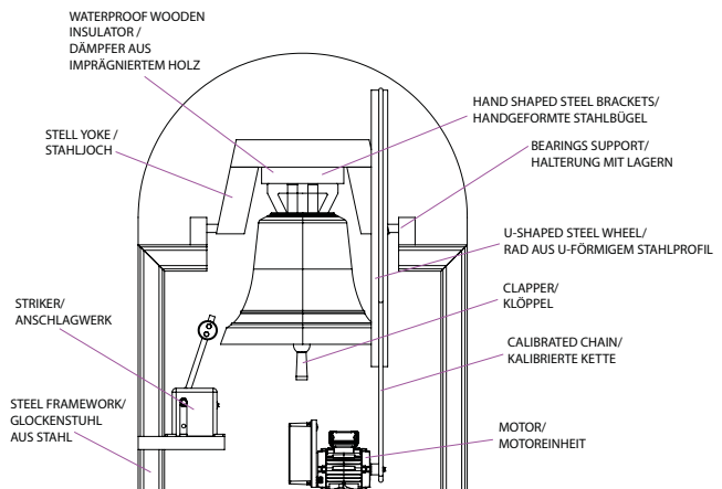
FALLING CLAPPER BELL GLOCKE MIT FALLKLÖPPEL
