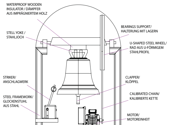
FLYING CLAPPER BELL GLOCKE MIT FLUGKLÖPPEL
